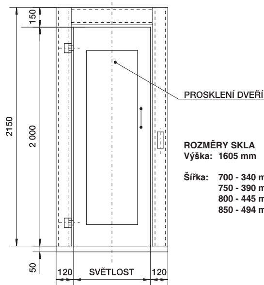
ŠACHETNÍ DVEŘE WIK - PANORAMATICKÉ SVĚTLOST VSTUPU: 700, 750, 800, 850, 900 PROVEDENÍ PRAVÉ, LEVÉ ( KRESLENO LEVÉ PROVEDENÍ )
